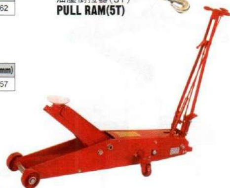
長型四輪千斤頂 LONG TYPE SERVICE JACK
